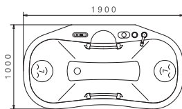
Dimensions Vis à Vis
